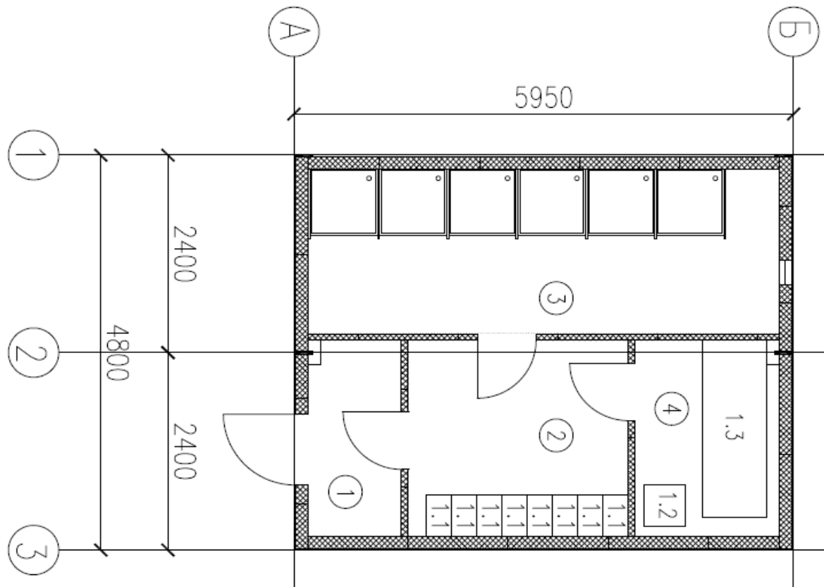
Модульное здание "Душевая"
